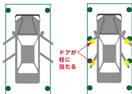
4本柱 スチールカーポートの場合
